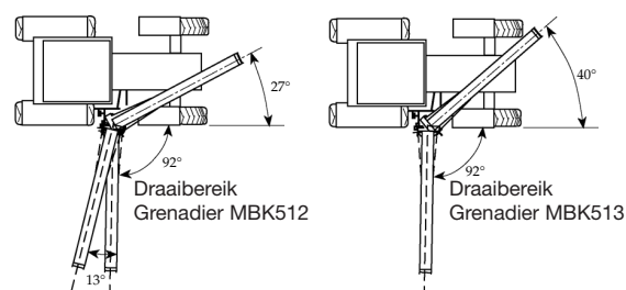
a) Werkbereik met maaikorf uit de draaikolom.
